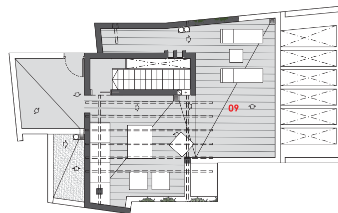
PLANTA SOLARIUM
