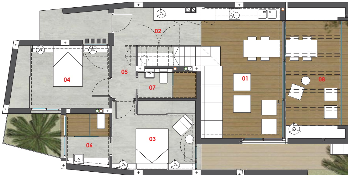
PLANTA PISO
