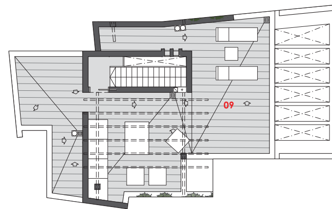
PLANTA SOLARIUM
