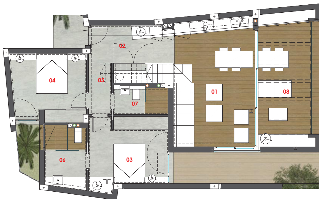
PLANTA PISO
