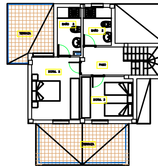
PLANTA PRIMERA
